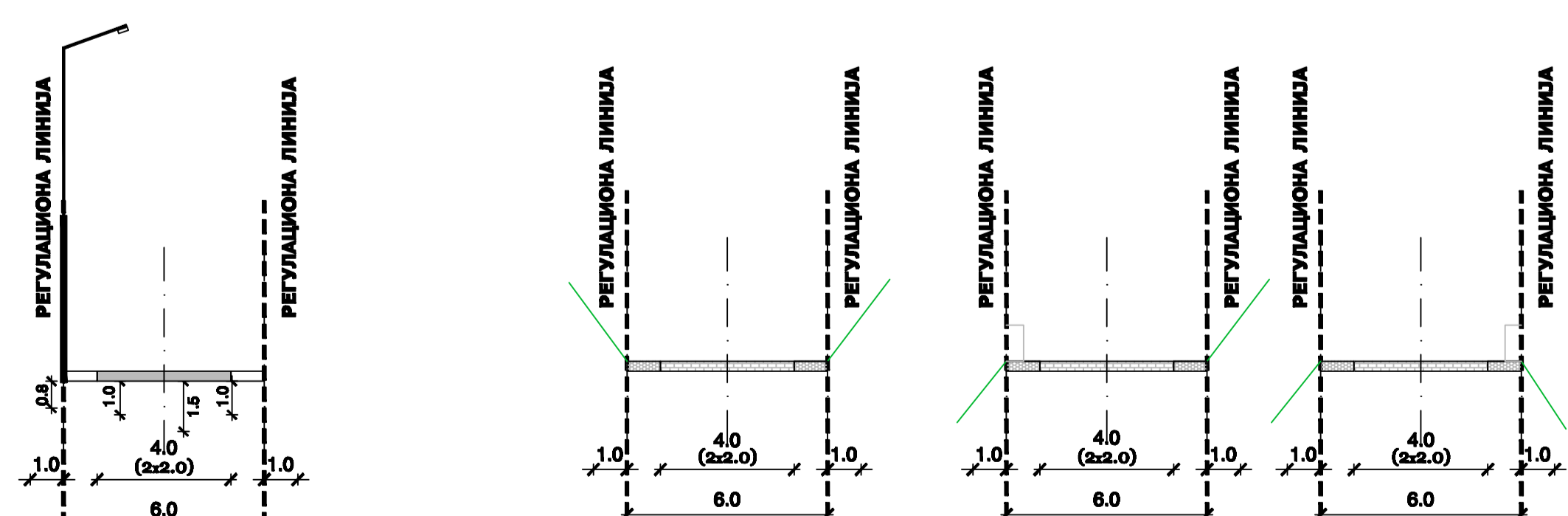
ПОПРЕЧНИ ПРОФИЛ 2-2
