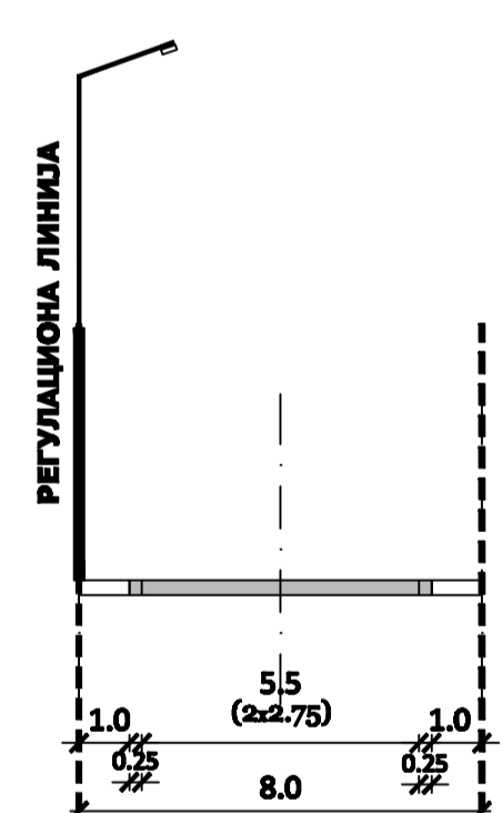
ПОПРЕЧНИ ПРОФИЛ 1-1
